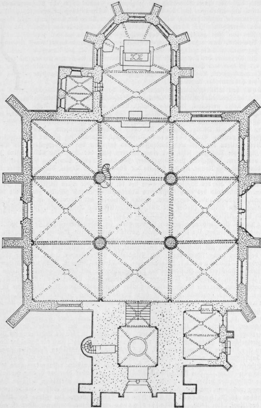
Abb. 58. Korbach, Grundriß der Milianskirche. 1 : 500
