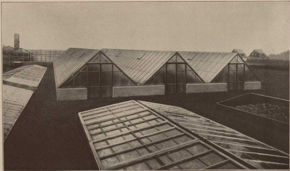
Gurkenhausanlage in kombinierter Holz- und Eisenkonstruktion für Gartenbaubetrieb Humig-Omsewitz
